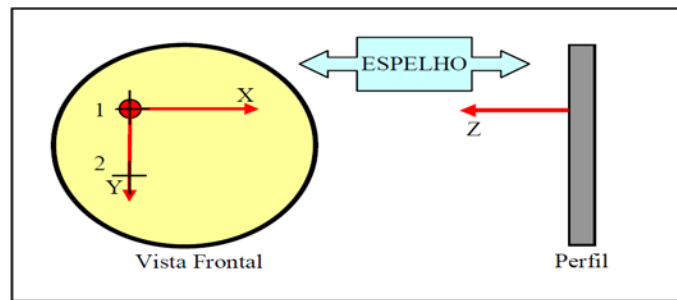
Figura 9 – Sistema de Eixos do Espelho.
