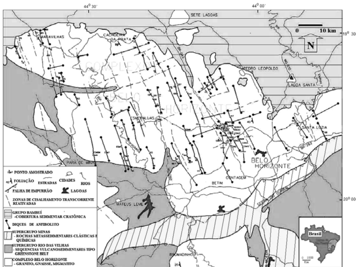
Figura 3 - Enxame Paraopeba de diques de anfíbolito no contexto geológico da porção meridional do Cráton São Francisco.
