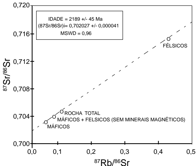
Figura 18 - Isócrona interna Rb-Sr para um anfibólito do enxame Paraopeba.
