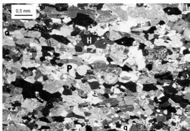
Figura 5 - Textura nematogranoblástica de uma amostra da porção marginal de um dique de anfibolito, sob nicóis cruzados. P = plagioclásio, H = hornblenda, A = augita, q = quartzo.
