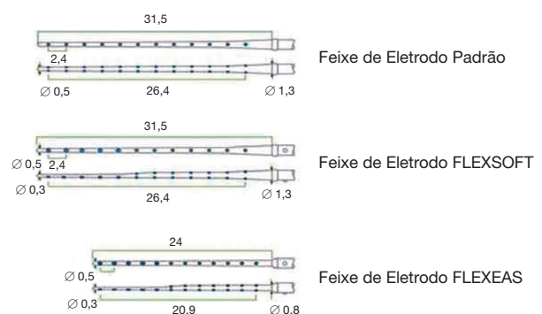
Figura 2 Esquema representativo do Eletrodo MED-EL FLEX™ EAS (21 mm).
