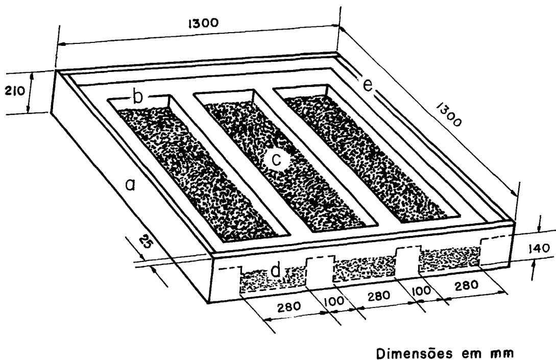
Figura 1. Coletor solar para desinfestação de substrato, com superfície absorvedora de chapa galvanizada ou chapa de alumínio.
