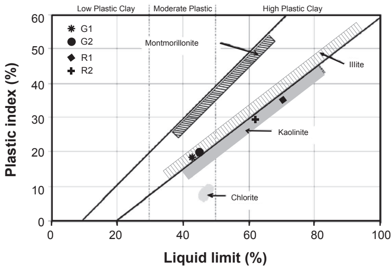
Figure 3: Position of clay samples on the Holtz and Kovacs diagram. [Figure 3: Posição das amostras de argila no diagrama de Holtz e Kovacs.]
