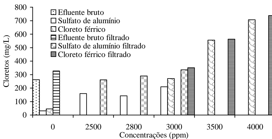
FIGURA 5: Caracterização dos valores de cloretos (mg/L) do efluente bruto não filtrado e filtrado, submetidos aos tratamento com sulfato de alumínio e cloreto férrico ambos não filtrado e filtrado.
