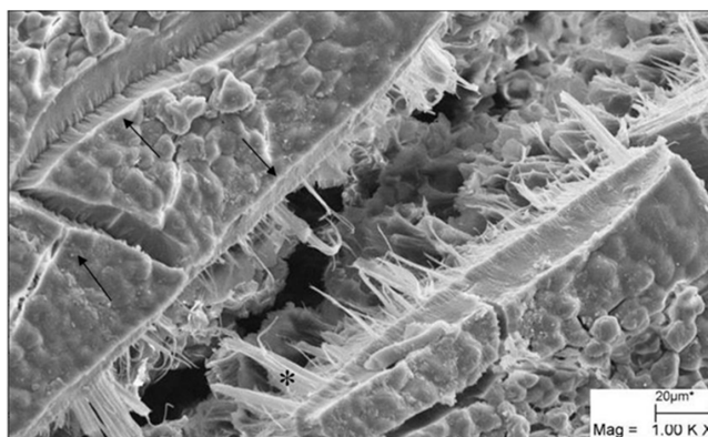
FIGURA 2: Eletromicrografia de varredura da testa de sementes de garapa, apresentando rachadura na testa (→), atingindo a camada de macroscleídes em paliçada (*), ocasionada pela água aquecida a 80°C por 30 segundos. UFV, Viçosa - MG.
