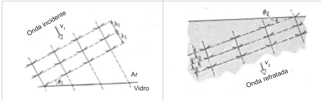
Figura 2. Ilustração do fenômeno de refração da luz, usando o Princípio de Huygens, no texto de Halliday/Resnick (1966, p. 1165 e 1995, p. 67).
