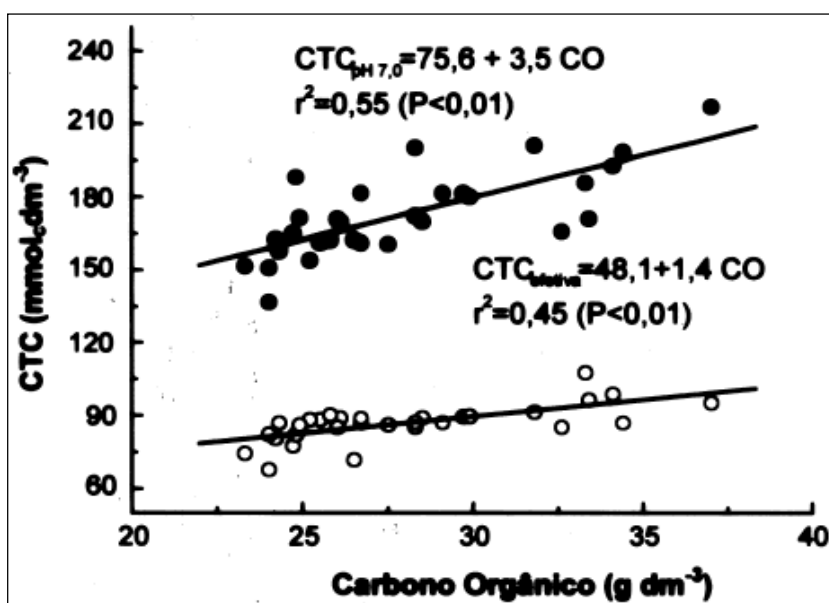
Figura 3 – Relação entre os teores de carbono orgânico e a capacidade de troca de cátions (CTC) a pH 7,0 e efetiva de um Latossolo Vermelho distroférico sob preparo reduzido. Cada ponto no gráfico representa uma profundidade do solo (0-2,5, 2,5-5, 5-7,5, 7,5-10, 10-15, e 15-20 cm) sob os diferentes sistemas de cultura, na média de três repetições.
