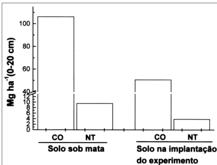
Figura 1 – Estoques de carbono orgânico (CO) e nitrogênio total (NT) na camada de 0-20cm de um Latossolo Vermelho distroférrico sob mata e na implantação do experimento, ou seja, após 23 anos de cultivo baseado em preparo intensivo do solo, com arações e gradagens.
