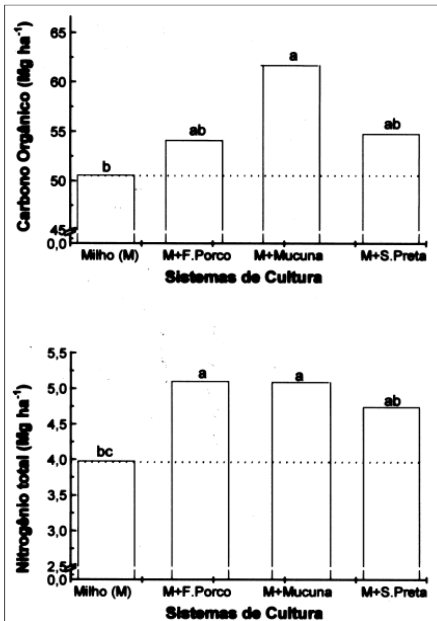
Figura 2 – Estoques de carbono orgânico e nitrogênio total na camada de 0-20 cm de um Latossolo Roxo distroférrico sob diferentes sistemas de cultura, em preparo reduzido durante cinco anos. Letras diferentes sobre as colunas indicam diferença significativa pelo teste de Tukey ao nível de 5%.
