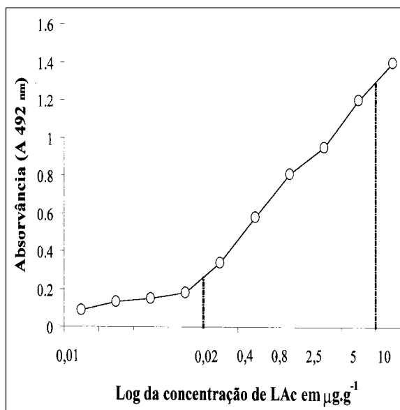
Figura 2 - Curva de calibração utilizada na quantificação de acetato de lupeol (LAc) através ELISA indireto. As absorvâncias a 492 nm foram relacionadas com valores em \text{ppm.mL}^{-1} correspondentes às diferenças entre as absorvâncias em extratos metanólicos de Vernonia scorpioides e o sistema branco (sem LAc). As linhas pontilhadas indicam os limites mínimo e máximo de detecção de LAc através de IgY-ELISA anti-Lac.
