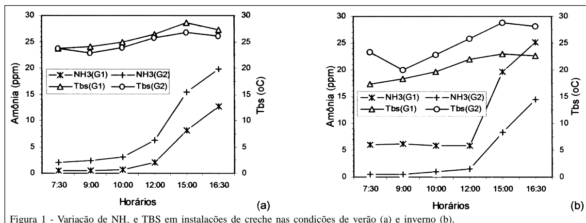
Figura 1 - Variação de NH 3 e TBS em instalações de creche nas condições de verão (a) e inverno (b).
