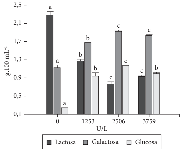
Figura 2. Concentraciones de lactosa, galactosa y glucosa ( \text{g} \cdot 100 \text{ mL}^{-1} ) en yogures con distintas dosis de \beta -galactosidasa (0, 1253, 2506 y 3759 U/L). Letras distintas indican diferencias significativas ( p \leq 0,05 ) para cada componente entre tratamientos.
