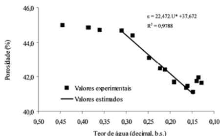
FIGURA 2 - Valores da porosidade calculados e estimados em função do teor de água dos grãos de soja
