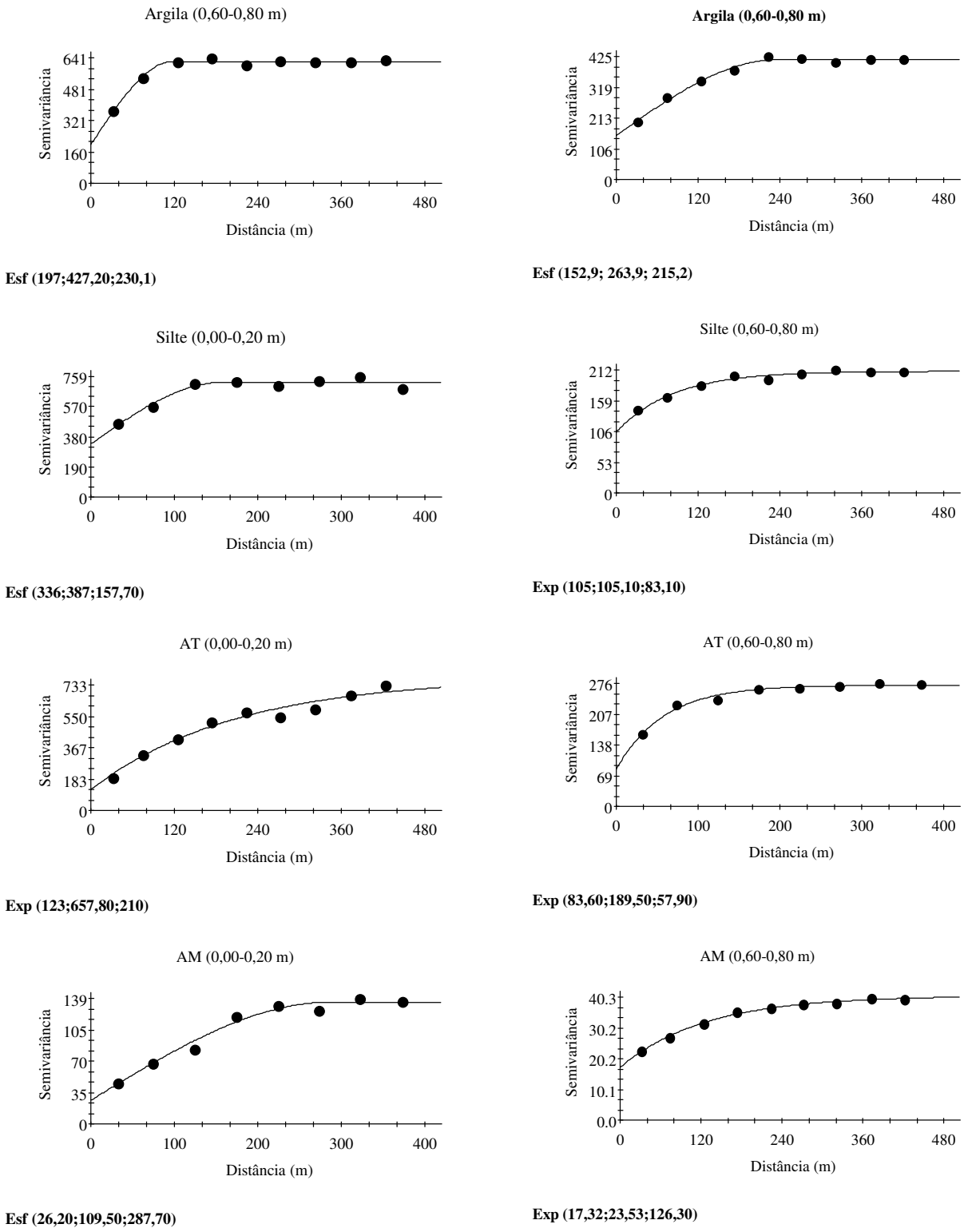
FIGURA 2. Semivariogramas das variáveis granulométricas argila, silte, areia total e areia média ( g\ kg^{-1} ) nas profundidades de 0-0,2 m e 0,6-0,8 m. Esf e Exp ( C_0; C_0+C_1; a ) são o modelo esférico e exponencial ajustado, C_0 = efeito pepita; C_0+C_1 = patamar; a = alcance.
