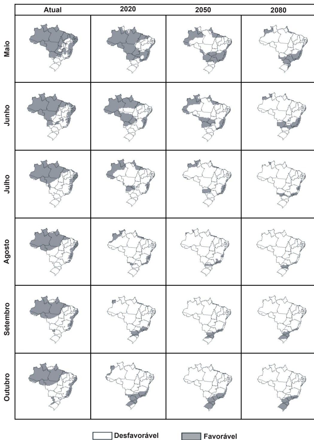
FIG. 2 - Mapa de favorabilidade climática à sigatoka-negra da bananeira no Brasil, para os meses de maio a outubro, no período atual (média de 1961 a 1990) e futuro (2020, 2050 e 2080, para o cenário A2).
