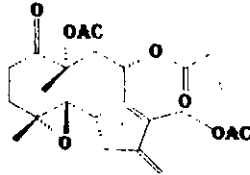
glaucolideo B isolado de V. eremophila com atividade moluscocida para ovos de B. glabrata (ALARCON, 1990).
