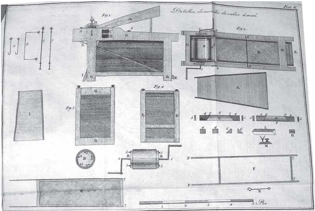
Figura 2: Moinho manual de despulpamento (Laborie, 1800)
