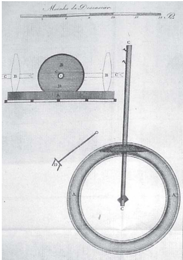
Figura 3: Moinho de descascar (Laborie, 1800)
