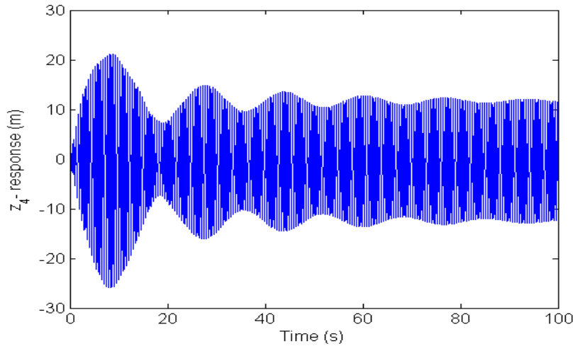
Fig. 5(b): Typical beat phenomenon.
