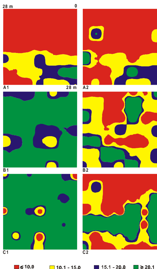
FIG. 2. Distribuição espacial dos valores de P do solo ( \text{mg dm}^{-3} ) nos diferentes sistemas de preparo e profundidade de amostragem (A: arado; B: grade; C: plantio direto; 1: 0-5 cm; 2: 5-20 cm de profundidade).
