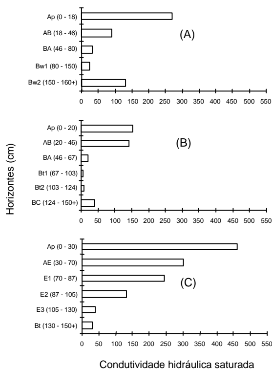
FIG. 2. Condutividade hidráulica saturada ( \text{m s}^{-1} \times 10^{-7} ) do Latossolo Amarelo argissólico (A), Argissolo Amarelo (B) e Argissolo Acinzentado (C) da toposeqüência de tabuleiro do Estado da Bahia.
