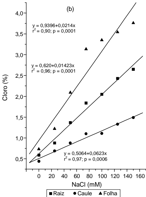
Figura 3. Porcentagem de cloro em raízes, caule e folhas de goiabeira em razão de níveis de NaCl na solução nutritiva após (a) 30 e (b) 50 dias de aplicação do estresse salino.
