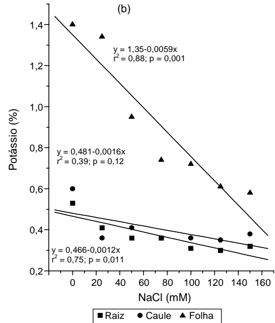
Figura 4. Porcentagem de potássio em raízes, caule e folhas de goiabeira em razão de níveis de NaCl na solução nutritiva após (a) 30 e (b) 50 dias de aplicação do estresse salino.
