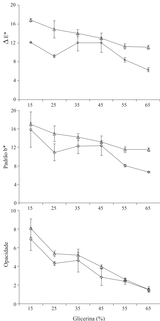
Figura 1. Diferença de cor ( \Delta E^* ), padrão b* e opacidade dos filmes com 1 (●) e 2 (△) g de proteínas do músculo de tilápia-do-nilo/100 g de solução filmogênica tratada a 90°C por 30 minutos, em razão da concentração de glicerina. As barras em cada ponto representam o desvio-padrão da média.
