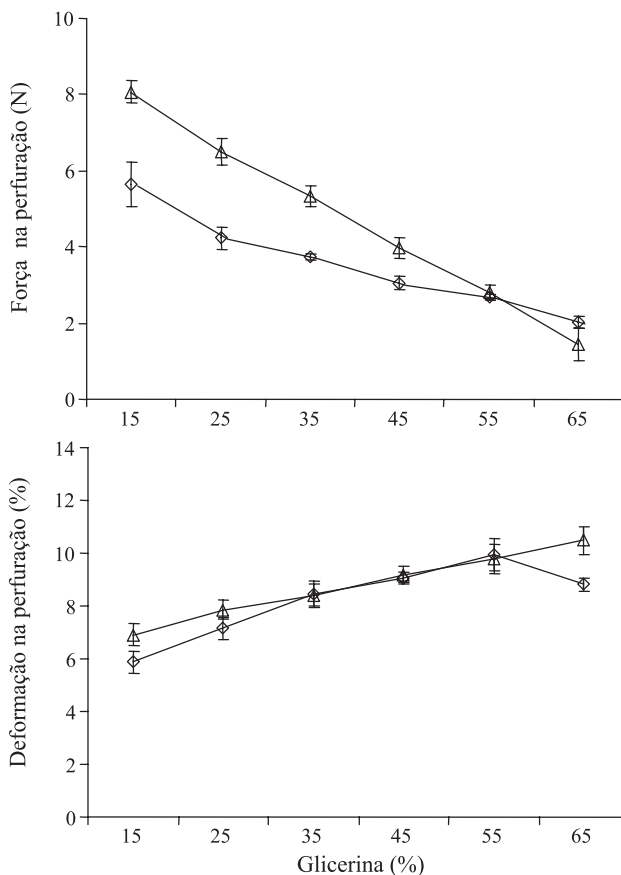
Figura 2. Força e deformação na perfuração dos filmes com 1 (●) e 2 (△) g de proteínas do músculo de tilápia-do-nilo/100 g de solução filmogênica tratada a 90°C por 30 minutos, em razão da concentração de glicerina. As barras em cada ponto representam o desvio-padrão da média.
