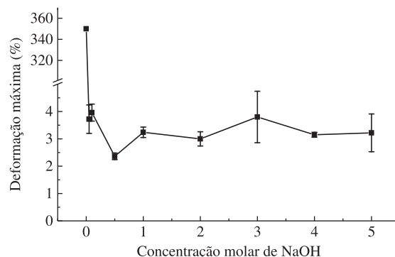
Figura 7. Propriedades tênsis do PET em função da concentração de NaOH a uma taxa de deformação de 5 mm/min.
