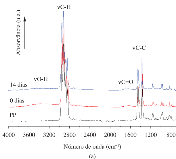
Figura 5. Espectros ATR-FTIR das amostras envelhecidas que foram tratadas por a) plasma e; b) VUV.
