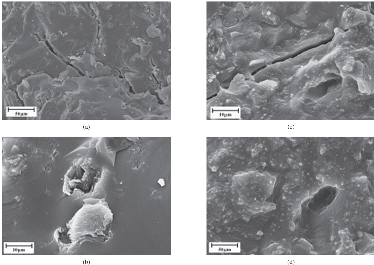
Figura 5. Imagens de MEV da superfície fraturada dos compósitos glioxal-fenol reforçado com (a), (b) 50% de CM (×1000, ×5000); (c), (d) 70% de CM (×3000, ×5000).
