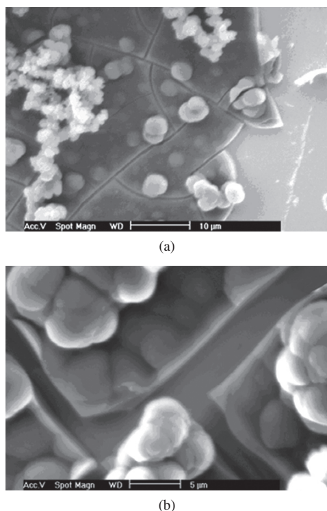
Figura 6. Micrografias de um filme de PAA formado sobre eletrodo de Pt pela aplicação de um potencial cíclico entre 0 e 600 mV/ECS durante 100 ciclos, num meio de 0,0025 M de 1-AA + HClO 4 com eletrodo de referência de calomelano saturado e contra eletrodo de platina.
