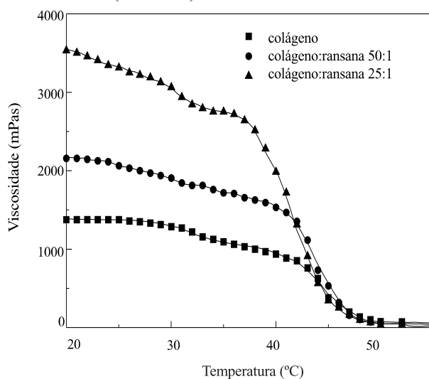
Figura 5. Efeito temperatura sobre a viscosidade de géis de colágeno:ransana determinadas em tampão fosfato, 0,13M, pH 7,4. Concentração de colágeno de 25 mg/g de gel.
