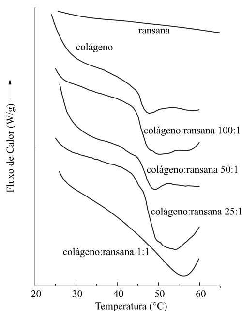
Figura 3. Calorimetria exploratória diferencial para membranas colágeno:ransana com concentrações variáveis do polissacarídeo, conformadas a pH 3,5.
