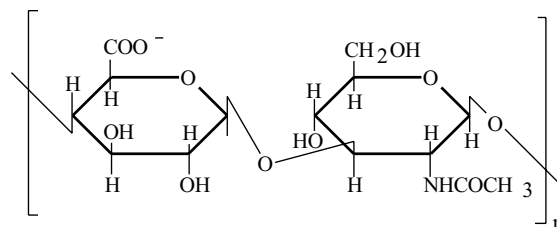
Figura 1. Estrutura da unidade repetitiva do ácido hialurônico.
