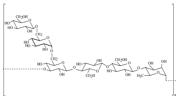
Figura 2. Estrutura primária de uma das cadeias da dupla hélice da ransana.
