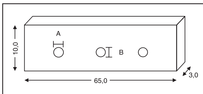
FIGURA 1 - Esquema representativo da amostra e medidas realizadas nas posições A e B.
