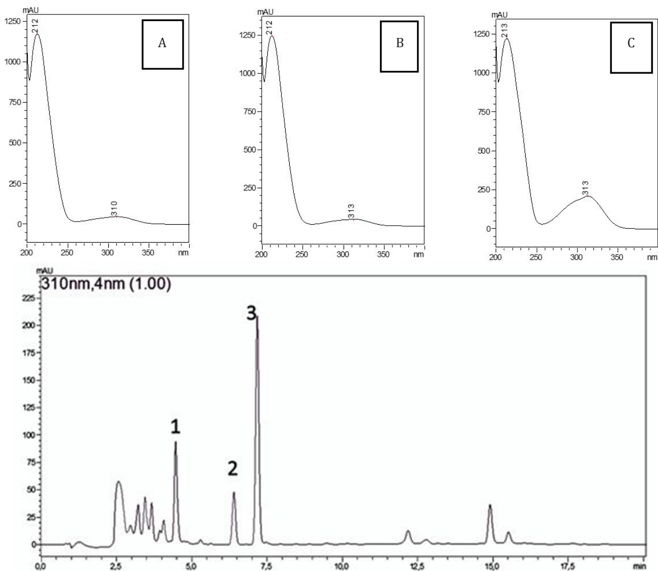
Fig.1. Cromatograma (HPLC-DAD em 310nm) do extrato etanólico bruto obtido das folhas de Hymenaea martiana Hayne. Em (A-C) constam três tipos de flavonoides que foram encontrado por HPLC-DAD, porém para sua identificação necessitam-se de maiores análises.
