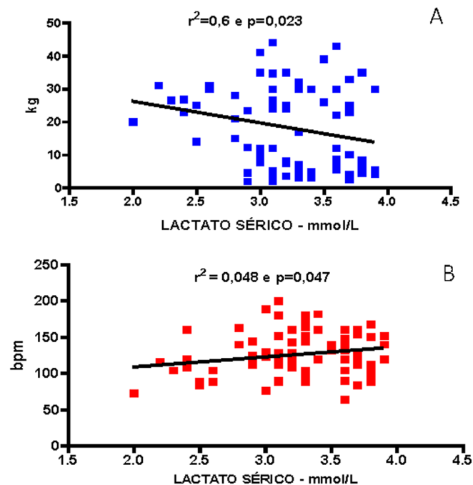
Fig.2. Representação gráfica da regressão linear dos valores de lactato sérico (valores expressos em mmol/L) em relação ao peso corporal (expresso em quilograma - kg) (A) e a frequência cardíaca em batimentos cardíacos por minuto (bpm) (B) de 80 cães saudáveis, avaliados durante o atendimento clínico ambulatorial veterinário.
