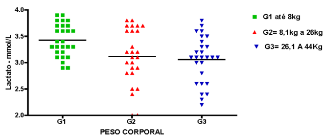
Fig.5. Representação gráfica dos valores referentes ao lactato sérico, obtidos em grupos de cães saudáveis (n=80) diferenciados conforme peso corporal expresso em quilograma (kg). G1 = até 8 kg; G2 = de 8,1 a 26 kg e G3 = de 26,1 a 44 kg, mensurado durante o atendimento clínico ambulatorial veterinário.
