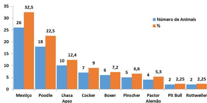
Fig.1. Distribuição racial de 80 cães saudáveis avaliados durante atendimento clínico ambulatorial, para a mensuração dos valores de lactato sérico.
