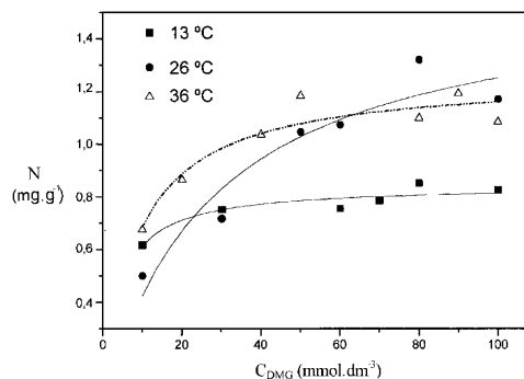
Figura 3. Isoterma de adsorção de Ni(II), das cápsulas adsorvidas com DMG; ( N = \text{massa de Ni(II)} \cdot \text{massa de cápsulas}^{-1} ).
