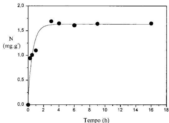
Figura 1. Cinética de adsorção de Ni(II), das cápsulas adsorvidas com DMG; ( N = \text{massa de Ni(II)} \cdot \text{massa de cápsulas}^{-1} ).
