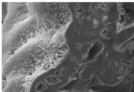
Figura 11. Micrografia da seção transversal da cápsula com o complexo Ni(DMG) 2 .
