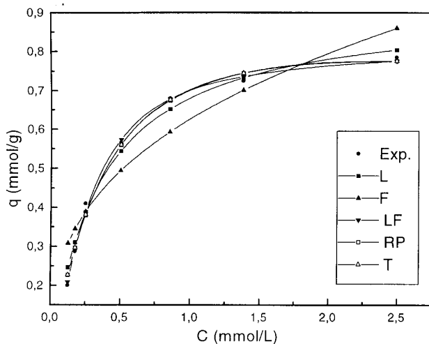
Figura 3. Ajustes dos dados experimentais de adsorção de Cu(II) com QTDH empregando as isotermas de Langmuir (L), Freundlich (F), Langmuir-Freundlich (LF), Redlich-Peterson (RP), Tóth (T).
