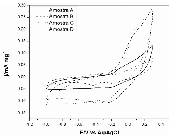
Figura 3. Perfis voltamétricos obtidos para eletrocatalisadores de Mn/C recuperados de pilhas usadas, em meio de NaOH 1 Mol L -1 . Velocidade de varredura de potenciais = 10 mV s -1 , E i -1 V e E f 0,25 V (vs. Ag/AgCl)
