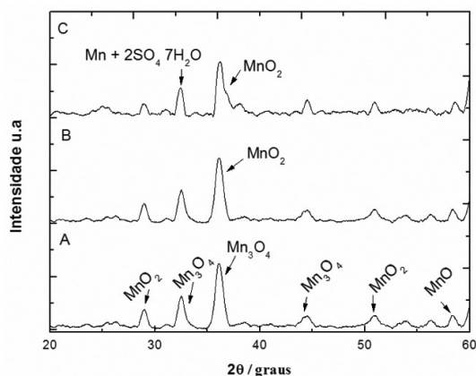
Figura 2. DRX das amostras: (1) Amostra A, (2) Amostra B e (3) Amostra C
