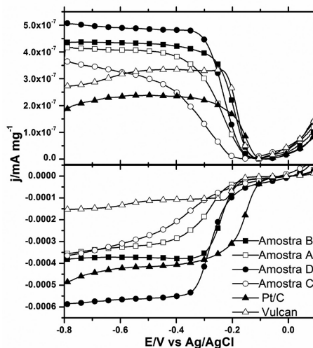
Figura 4. Curvas de polarização em estado estacionário para os diferentes eletrocatalisadores de Mn/C recuperados de pilhas usadas, em meio de NaOH 1 Mol L -1 : (a) corrente do anel e (b) corrente no disco. \omega = 1600 rpm. A curva de Pt/C foi inserida para comparação. Potencial do anel = 0,15 V
