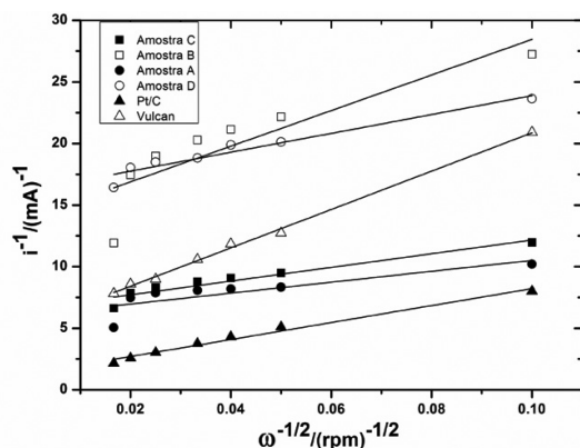
Figura 5. Diagrama de Koutecky-Levich para os eletrocatalisadores de Mn/C recuperados de pilhas usadas, em -0,22 V e solução de NaOH 1 Mol L -1 . Os valores de Pt/C e carbono Vulcan foram inseridos para comparação
