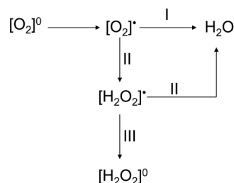
Figura 1. Esquema do mecanismo de reação de redução do oxigênio
