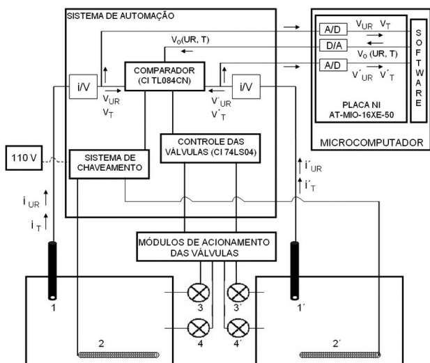
Figura 3. Diagrama esquemático do interfaceamento entre as câmaras e o microcomputador, 1 e 1': sensores de T e UR; 2 e 2': resistências internas; 3 e 3': válvulas solenoides de ar seco; 4 e 4': válvulas solenoides de ar úmido; i_{UR} e i'_{UR} correntes associadas aos sinais de UR medidos nas câmaras; i_T e i'_T correntes associadas aos sinais de T medidos nas câmaras; V_{UR} e V'_{UR} potenciais associados aos sinais de UR medidos nas câmaras; V_T e V'_T potenciais associados aos sinais de T medidos nas câmaras; V_0(UR, T) : potenciais associados aos valores de UR e T definidos para as câmaras pelo software; A/D: conversor analógico-digital; D/A: conversor digital-analógico
