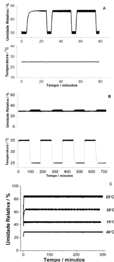
Figura 5. (A) Valores de UR e de T monitoradas na câmara de envelhecimento durante ciclos de UR entre 30% (5 min) e 80% (20 min) a 25 °C; (B) Valores de UR e de T monitorados na câmara de envelhecimento durante ciclos de T entre 25 °C (90 min) e 35 °C (90 min). (C) Valores máximos de UR alcançáveis na câmara de envelhecimento nas T de 25, 30, 35 e 40 °C
