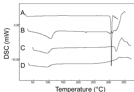
Figure 2. Thermograms of: (A) GEN; (B) \beta -CD; (C) GEN/ \beta -CD physical mixture and (D) GEN: \beta -CD complex
