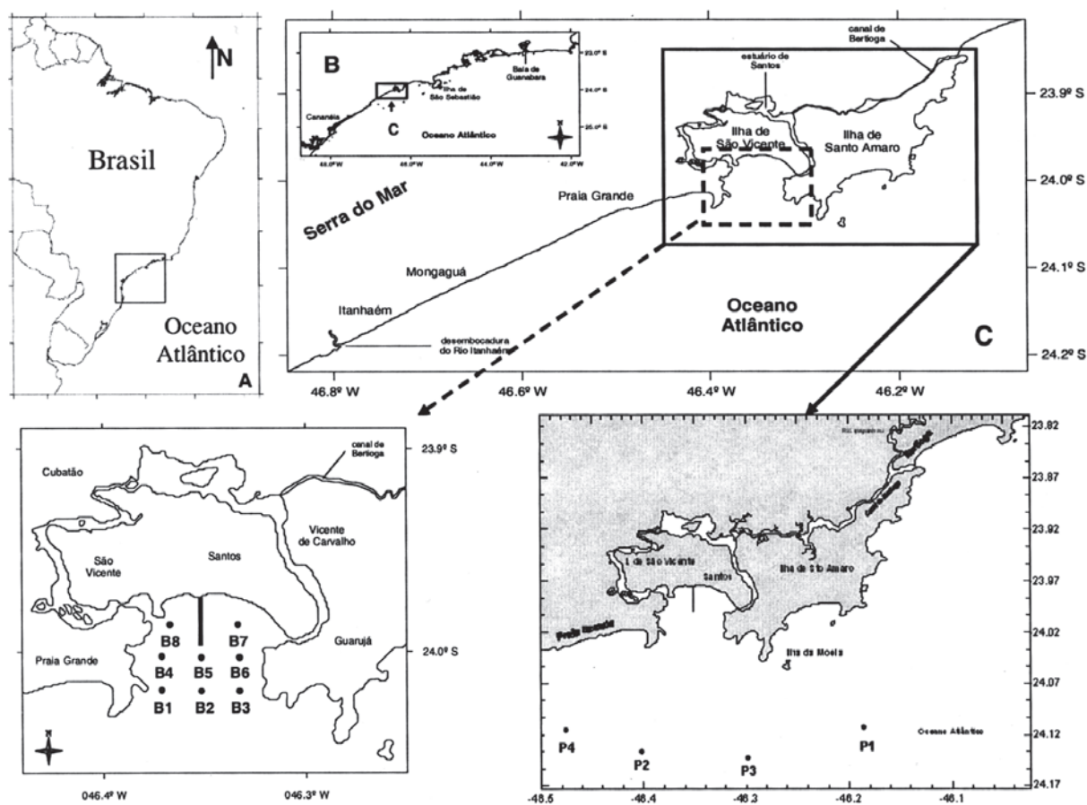
Figura 1S. Mapa da área de estudo e pontos de coleta de sedimentos. (A) Estado de São Paulo; (B) Baixada Santista; Baía de Santos e Plataforma Continental (C)
