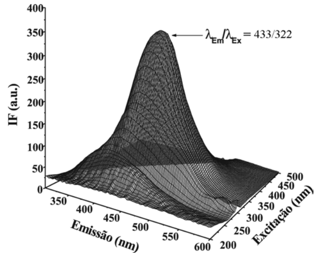
Figura 3. Espectro 3D da amostra de ácido fúlvico extraído da água (AF-LP)
