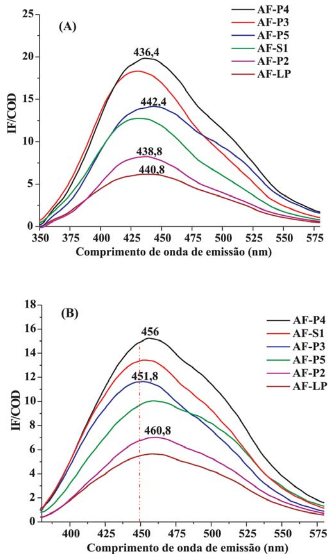
Figura 3S. Espectros de emissão (u.a.) dos ácidos fúlvicos com excitação em 314 (A) e 370 nm (B) normalizados pelo COD ( \text{mg L}^{-1} )
