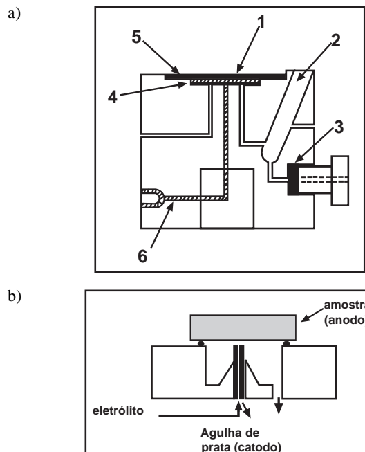
Figura 1. Células de eletrodissolução anódica: (a) original proposta por Bergamin et al 12 : 1 - célula eletrolítica, 2 - dispositivo para remover bolhas, 3 - unidade de filtragem, 4 - catodo (disco de latão recoberto com ouro), 5 - disco de borracha, 6 - contato elétrico; b) proposta por Souza et al 1,27 (alta densidade de corrente).
