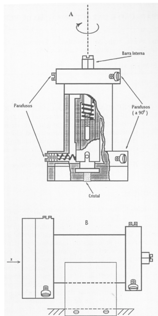
Figura 1. (a) Suporte em alumínio (corpo) e aço inoxidável (base) confeccionado para o polimento dos eletrodos monocristalinos, (b) Representação esquemática do suporte de polimento no banco óptico do equipamento de raios X.
