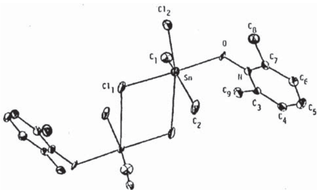
Figura 5. Estrutura do dímero de dicloreto de dimetilstanho(IV).2,6-dimetilpiridina.
