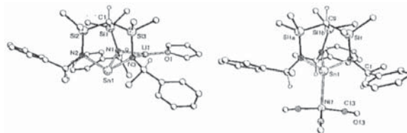
Figura 27. As estruturas do complexo quiral. [HC{SiMe 2 N[(S)-CH(Me)Ph]} 3 Sn] e de seu derivado heterobimetálico com o grupo Ni(CO) 3 .
