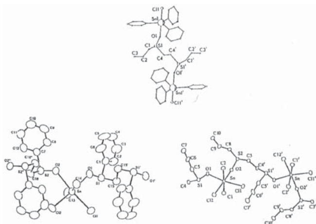
Figura 8. Estruturas do monômero com átomos de Sn pentacoordenados, [\text{Ph}_3\text{SnCl}\{\mu\text{-PrSOCH}_2\text{CH}_2\text{SOPr}\}\text{ClSnPh}_3] , e dos polímeros com átomos de Sn hexacoordenados, [\text{Me}_2\text{SnCl}_2(\text{PrSOCH}_2)_2]_n e [\text{Me}_2\text{SnCl}_2(\text{PhSOCH}_2)_2]_n .
