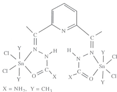
Figura 32. Fórmula molecular proposta para o complexo [(\text{Me}_2\text{SnCl}_2)_2(\text{H}_2\text{dapsc})] .
