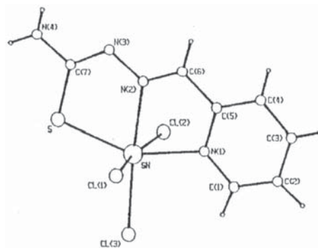
Figura 30. Estrutura do complexo [SnCl_3(FPT)] .
