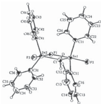
Figura 9. Estrutura do complexo [(\text{Ph}_2\text{FSn})_2\text{CH}_2\text{F}]^- .
