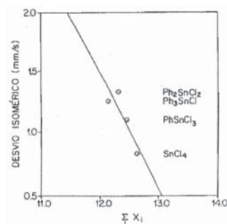
Figura 15. Gráfico de desvio isomérico contra \Sigma_i X_i onde X = eletronegatividade de Pauling do ligante i.
