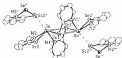
Figura 19. Estrutura do complexo heterocatenado dimérico [Sn(2-SeNC 5 H 4 ) 2 ] 2 .
