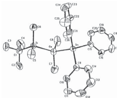
Figura 18. Estrutura do complexo heterocatenado [Me 2 CSiMe 2 GeMe 2 SnPh 3 ].
