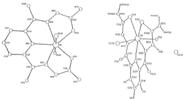
Figura 31. Estruturas dos complexos heptacoordenados (\text{MeSnCl}(\text{Hdaptsc}))\text{Cl}\cdot\text{MeOH} e [\text{MeSnCl}(\text{H}_2\text{dapsc})]\text{Cl}_2\cdot 2\text{H}_2\text{O} .
