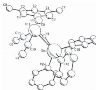
Figura 26. Estrutura do complexo bimetalico. [(η 6 -1,3,5-Me 3 Ph)(CO) 2 Cr(H)SnPh 3 ] com um ligante H coordenado de forma η 2 aos átomos de Cr e Sn.
