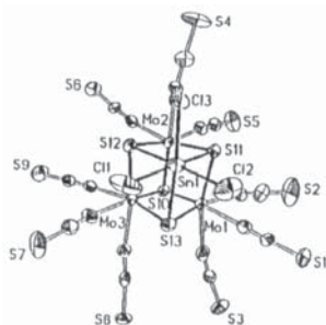
Figura 22. O cluster cúbico [Mo_3(SnCl_3)S_4(NCS)_9]^{5-} .
