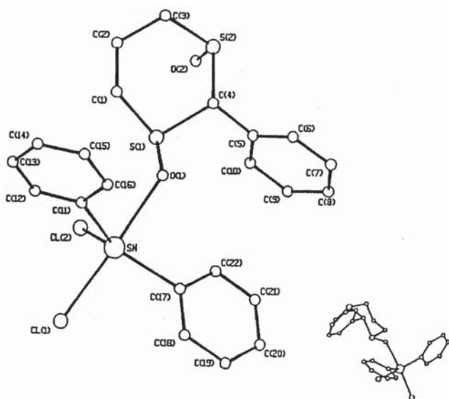
Figura 3. Estrutura molecular do aduto monomérico pentacoordenado [\text{Ph}_2\text{SnCl}_2 \cdot \text{CH}_2(\text{CH}_2)_2\text{SOCH}(\text{Ph})\text{SO}] .
