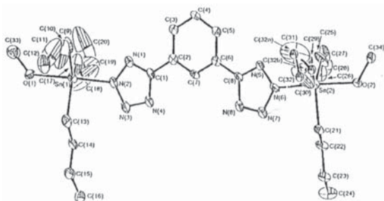
Figura 28. Exemplo de composto supramolecular do tipo bis(organoestânio)tetrazol com ponte de fenileno.
