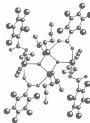
Figura 33. Estrutura do complexo dimérico bis(perfluorobenzoato)tetra-n-butilestanoxano.
