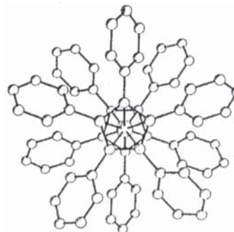
Figura 12. A estrutura do decafenilestanoceno, [(\eta^5\text{-}(\text{Ph})_5\text{C}_5)_2\text{Sn}(\text{II})] , vista perpendicularmente aos planos dos anéis ciclopentadienila.
