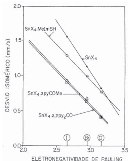
Figura 14. Gráfico de desvio isomérico contra a eletronegatividade de Pauling dos halogênios em SnX 4 , e em três famílias SnX 4 .L.
