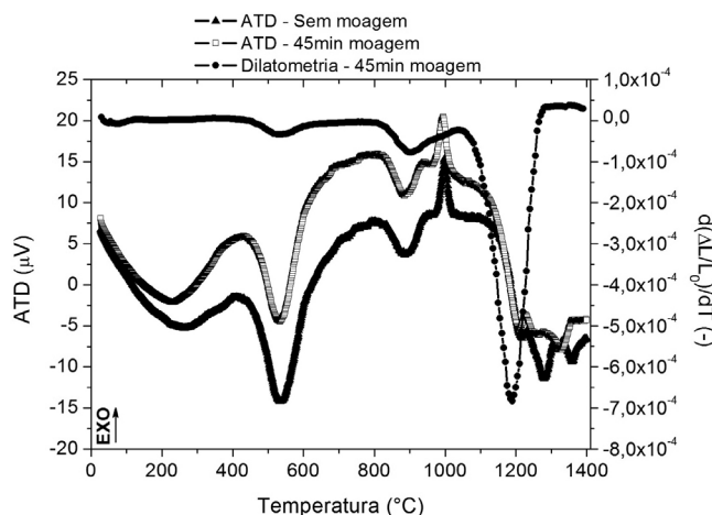
Figura 2. Resultados de ATD da formulação in natura e curvas de ATD e dilatometria após 45 min de moagem
