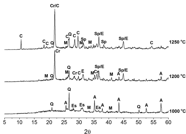
Figura 6. Difratomogramas de raios X das amostras da formulação moída por 45 min, tratadas por uma hora, em função da temperatura de tratamento. A: \alpha -alumina; C: \alpha -cordierita; Cr: cristobalita; E: Espinélio; Es: enstatita; M: mulita; Q: \alpha -quartzo; Sp: safirina
