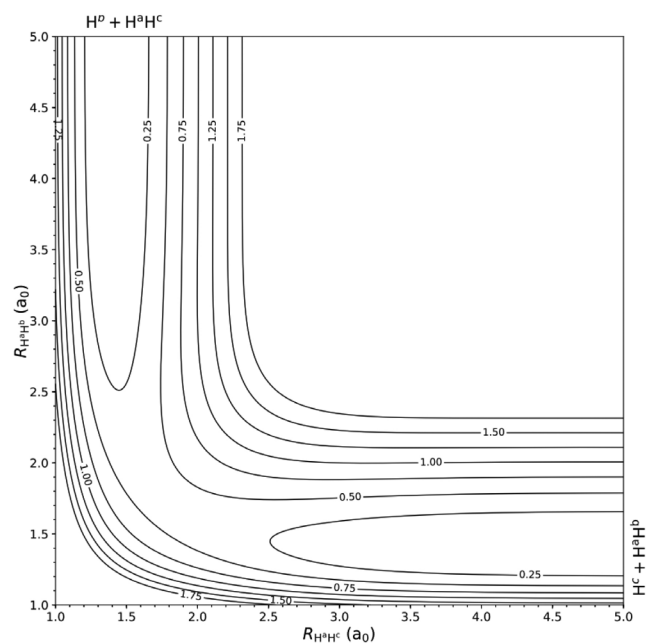
Figura 3. SEP da reação H^a + H^b H^c \rightarrow H^b + H^a H^c colinear, ajustada pela rede neural, em coordenadas internas ( R_{H^a H^c} , R_{H^a H^b} ). As curvas isopotenciais são de 0,25 eV. As distâncias, nos dois eixos, estão em a_0
