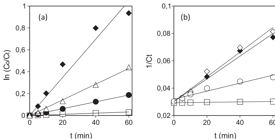
Figura 2. Curvas obtidas para a descoloração do corante vermelho de fenol a partir do modelo de 1ª ordem (a) por: \text{Fe}^{3+}/\text{H}_2\text{O}_2 ( \square ), \text{Fe}^{3+}/\text{H}_2\text{O}_2 /catecol ( \bullet ), \text{Fe}^{3+}/\text{H}_2\text{O}_2 /ácido 3,4-DHFA ( \triangle ) e \text{Fe}^{3+}/\text{H}_2\text{O}_2 /ácido 2,5-DHB ( \blacklozenge ); e a partir do modelo de 2ª ordem (b) por: \text{Fe}^{3+}/\text{H}_2\text{O}_2 ( \square ), \text{Fe}^{3+}/\text{H}_2\text{O}_2 /ácido gálico ( \circ ), \text{Fe}^{3+}/\text{H}_2\text{O}_2 /ácido 2,5-DHB ( \blacklozenge ) e \text{Fe}^{3+}/\text{H}_2\text{O}_2 /ácido 2,3-DHB ( \diamond ). [\text{H}_2\text{O}_2] = 450 \mu\text{mol L}^{-1} ; [\text{corante}] = 30 \mu\text{mol L}^{-1} ; [\text{mediador fenólico}] = 10 \mu\text{mol L}^{-1} ; \text{pH} = 2,5-3,0
