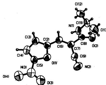
Figura 2. Conformación molecular del compuesto C_{11}H_{11}N_3O_4 .
