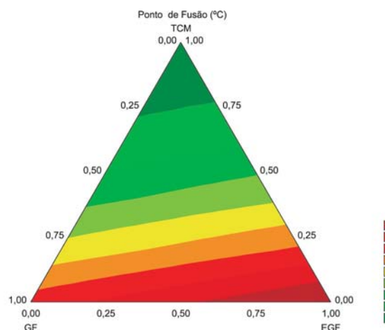
Figura 6. Diagrama triangular do ponto de fusão para os lipídios estruturados. Gordura abdominal de frango (GF) Estearina (EGF) Triacilgliceróis de cadeia média (TCM)
