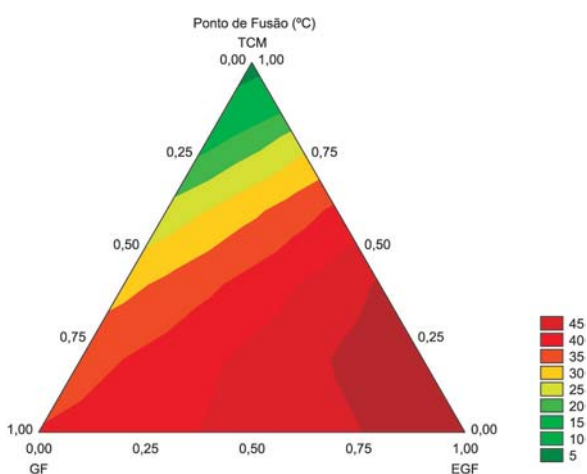
Figura 4. Diagrama triangular do ponto de fusão das amostras individuais e para as misturas binárias e ternárias da gordura abdominal de frango (GF), sua estearina (EGF) e triacilgliceróis de cadeia média (TCM)
