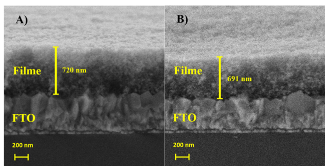
Figura 4. Imagem de MEV de secção transversal de filme de \text{TiO}_2 feito em spin coater : a) artesanal e b) comercial
