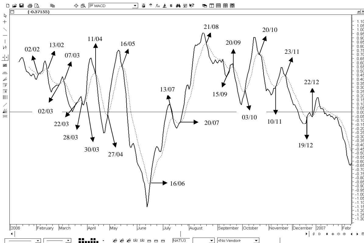
Figura 5: MACD (NATU3)
