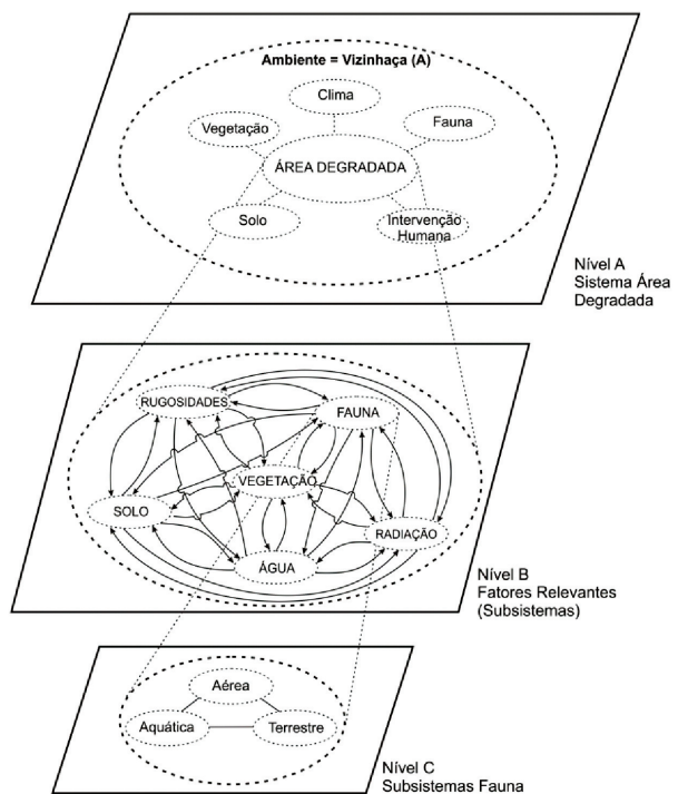
Figura 1 – Diagrama simplificado do sistema degradado com os componentes do ambiente (nível A). No nível B estão representados os elementos (subsistemas) da área degradada e no nível C estão representados os componentes do subsistema da fauna.
