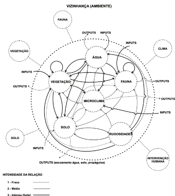
Figura 2 – Concepção do modelo de sistema ecológico para recuperação de um ecossistema degradado.
