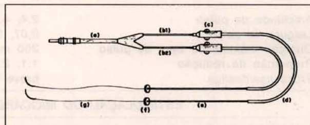
Fig. 5 - Esquema do eletrodo de implantação muscular modelo CM60-BP (Biotronic). (a) Conexão do eletrodo com o mioestimulador. (b1) Catódo. (b2) Ânodo. (c) Fixadores da capa móvel de silicone. (d) Capa móvel de silicone. (e) Eletrodo. (f) Discos de silicone. (g) Fio de Polipropileno 3.0 com agulha.
