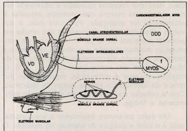
Fig. 4 - Esquema demonstrativo do funcionamento do cardiomiostimulador Myos (Biotronic)
