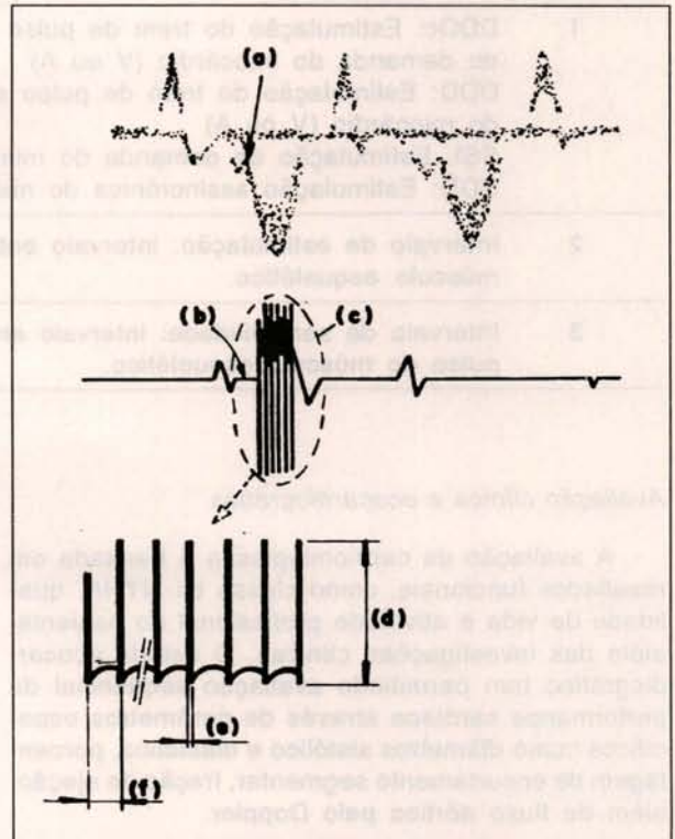
Fig. 7 - Esquema do sincronismo da estimulação muscular com a abertura da valva aórtica. (a) Abertura da valva aórtica. (b) Atraso da estimulação sincronizada com a abertura da valva aórtica. (c) Estimulação elétrica do músculo grande dorsal. (d) Amplitude de pulso. (e) Largura de pulso. (f) Intervalo de pulso.
