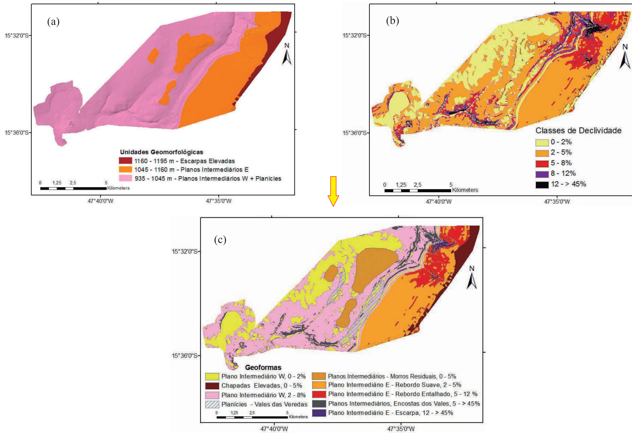
Figura 2. Mapa de unidades geomorfológicas (a), mapa de classes de declividade, ambos gerados a partir do MDT (Modelo Numérico do Terreno) (b), e mapa de geomorfias da Estação Ecológica de Águas Emendadas, DF (c), produto do cruzamento-soma dos mapas de unidades geomorfológicas e de classes de declividade.
